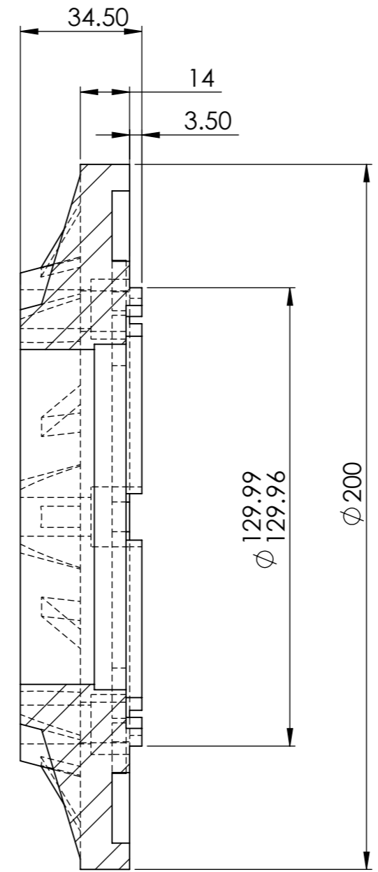
SECTION A-A
