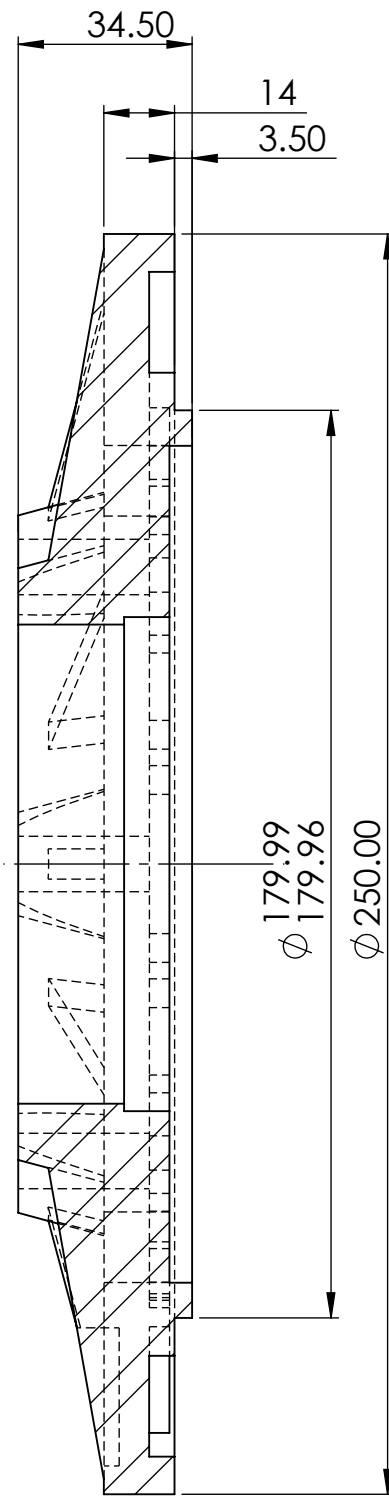
SECTION A-A
