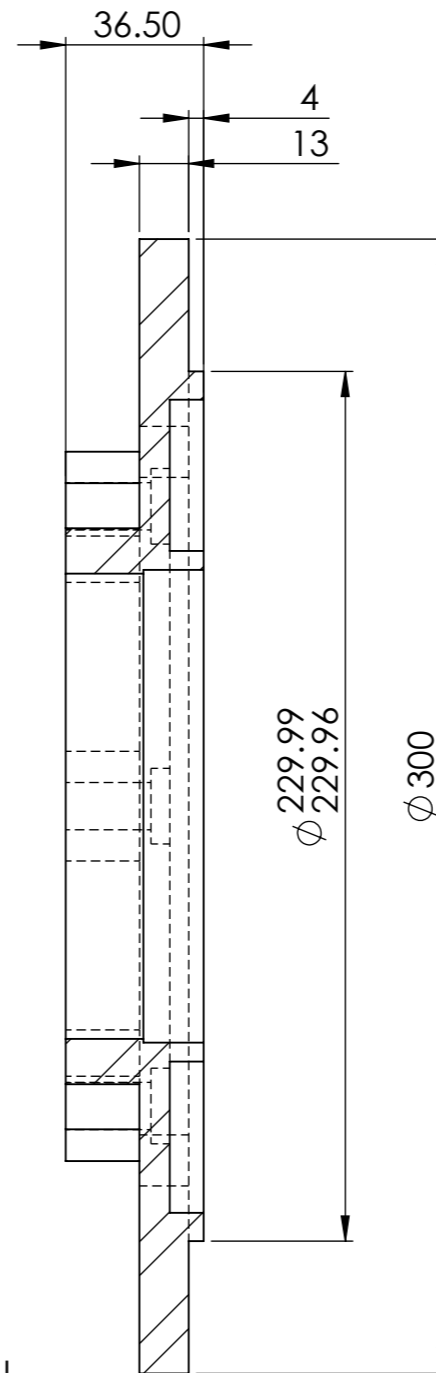
SECTION A-A
