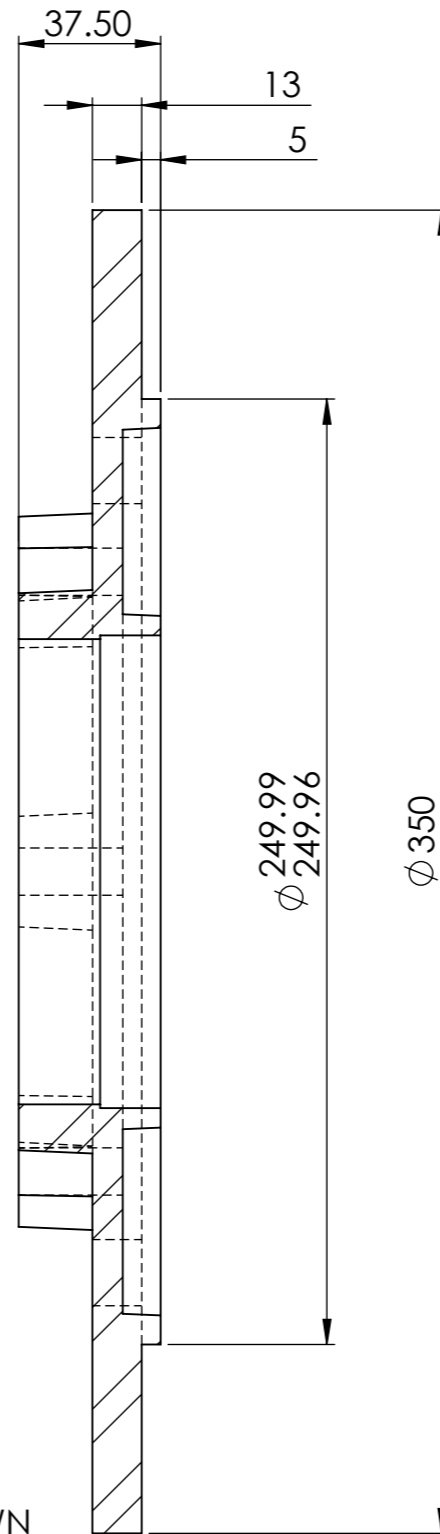
SECTION A-A
